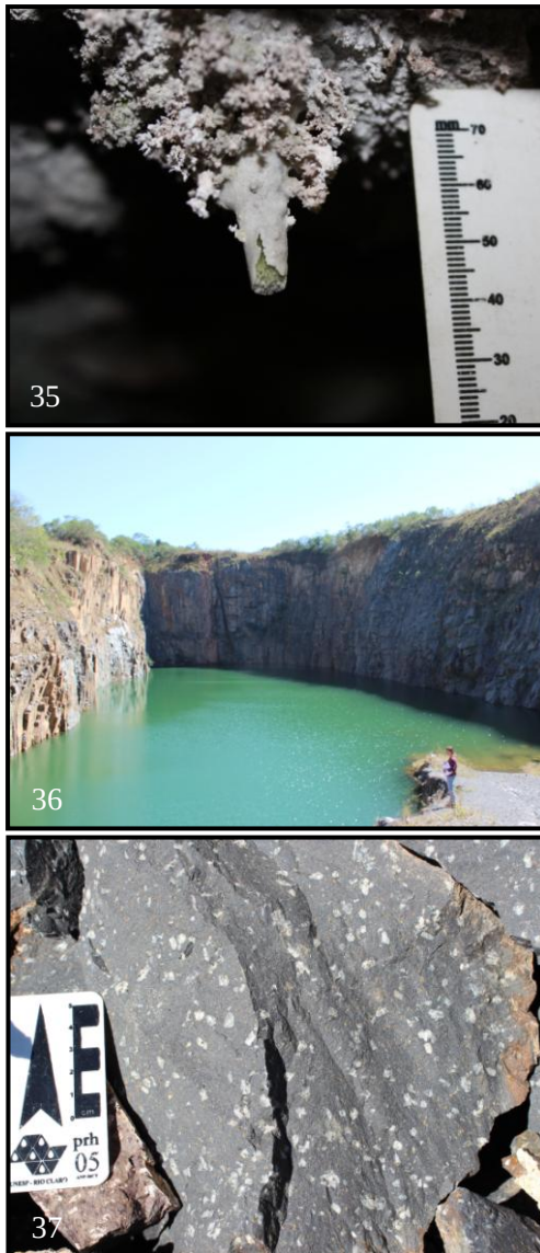
Figura 35 – Espeleotema carbonático do tipo “canudo” na gruta Casa de Pedra. Foto: HSP; Figura 36 – Pedreira Fortaleza. Na esquerda da foto: disjunções colunares na parede da pedreira. Foto: HSP; Figura 37 – Dacito com cristais de feldspato. Foto: HSP.
