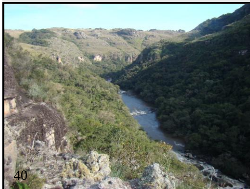
Figura 38 – Diamantes provenientes de uma área de mineração ativa em Tibagi. Foto: GBG; Figura 39 – Cenário retratando um acampamento de garimpeiros no Museu do Garimpo. Foto: NFM; Figura 40 – Canyon do Guartelá ou canyon do rio Iapó Foto: GBG.
